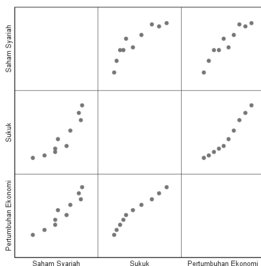
Gambar 3. Grafik Scatter plot
